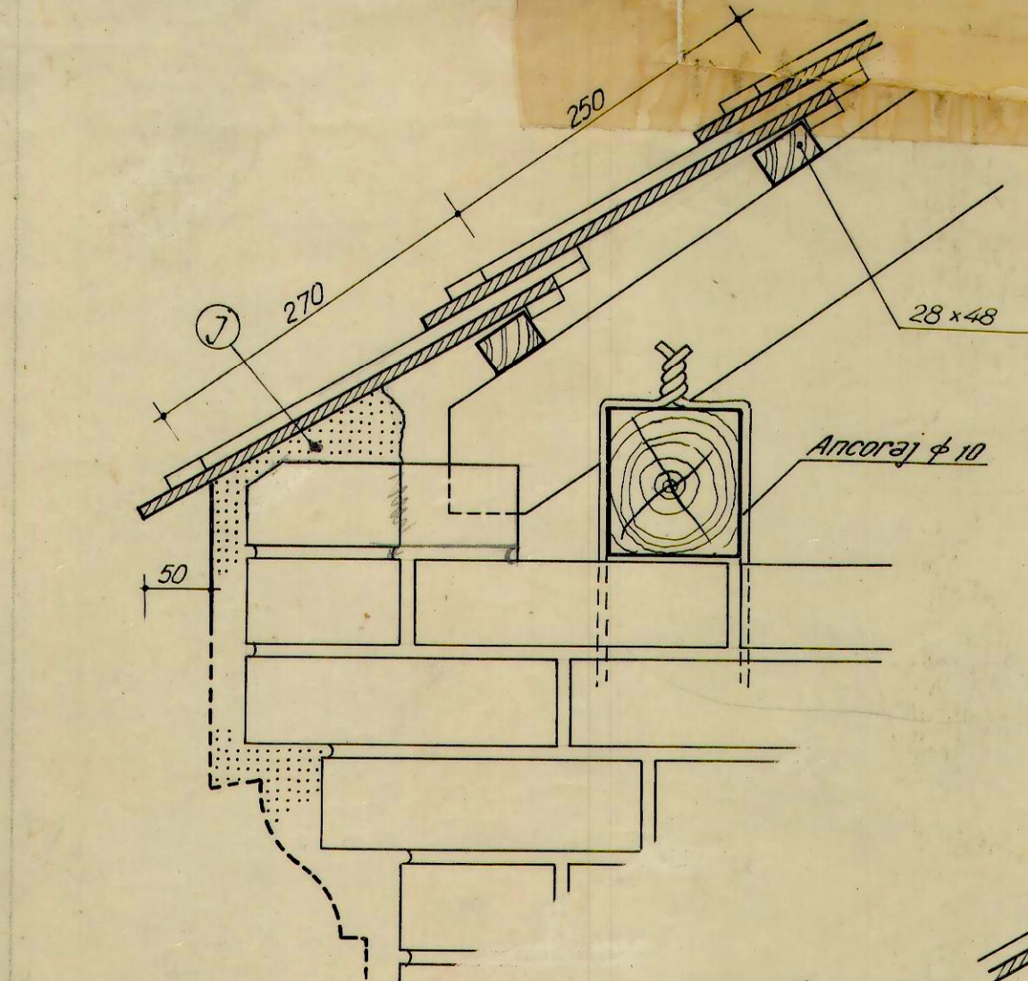
1 CORNISE ZIDITĂ
