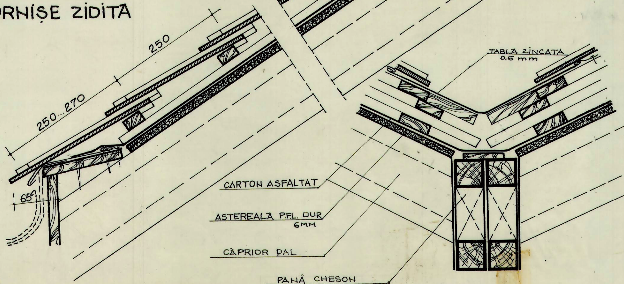
② STREĂȘINA
