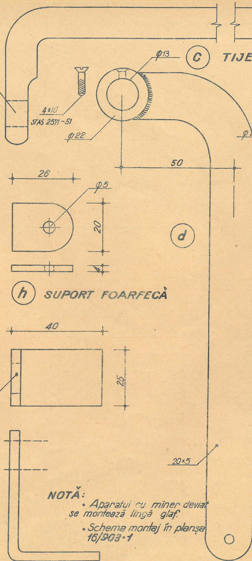
(f) SUPORT TIJĂ
