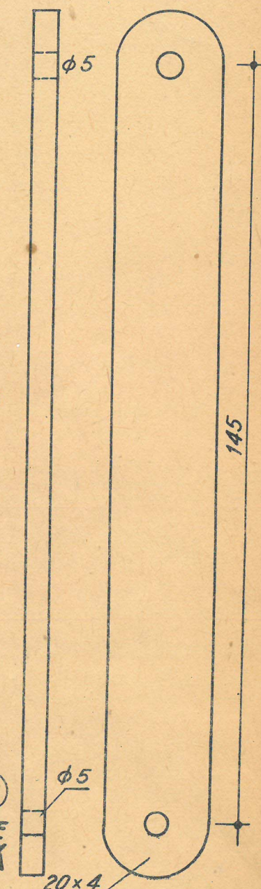
PRINDERE FOARFECĂ
