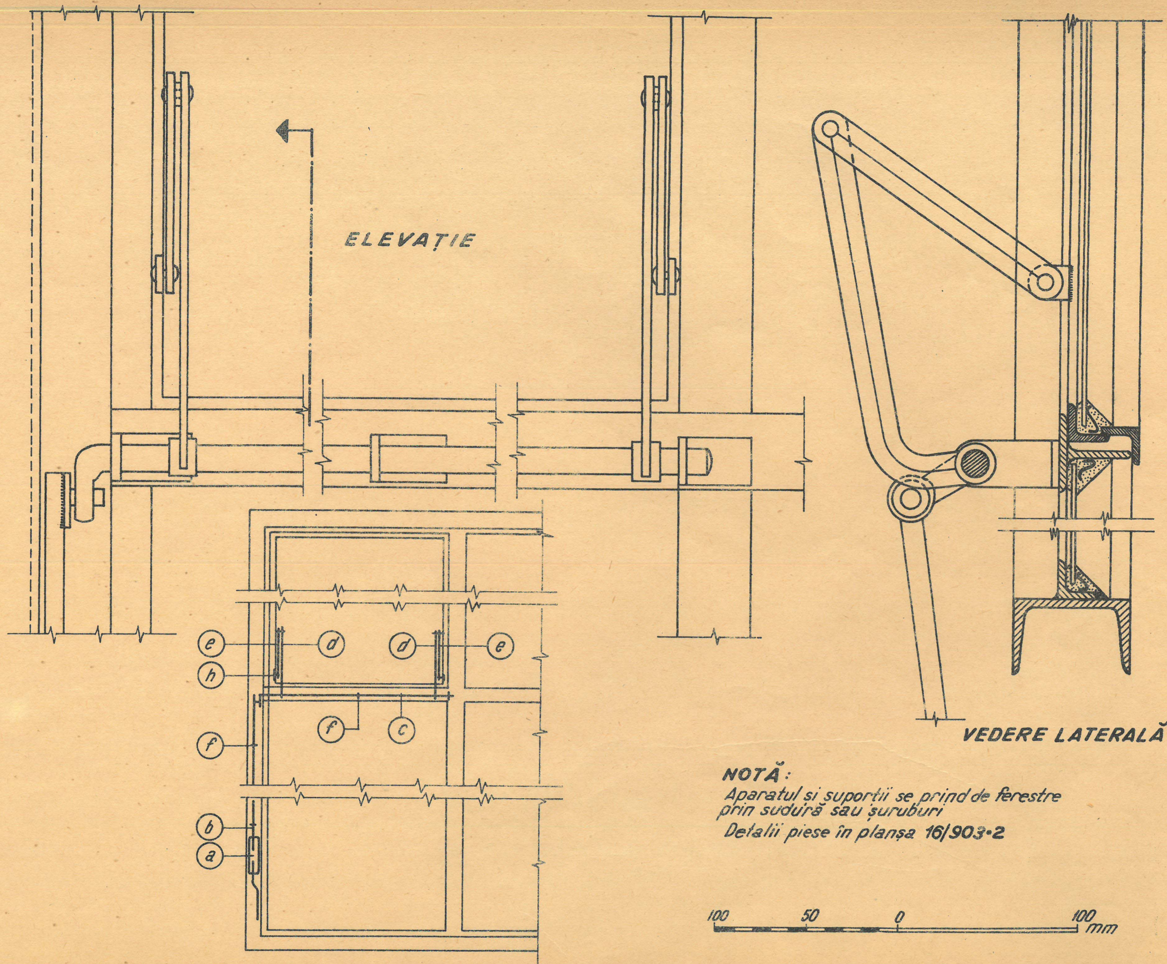
SCHEMA DE MONTAJ
