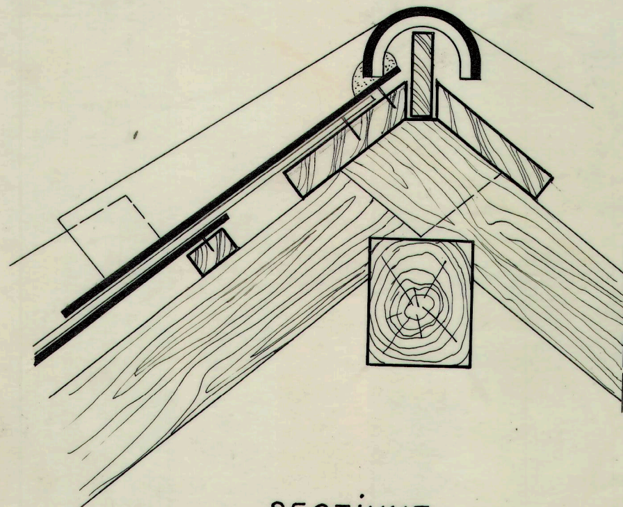
SECȚIUNE
