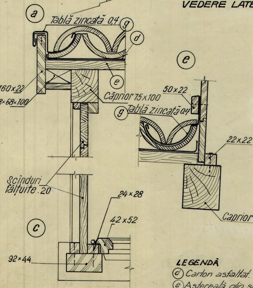
VEDERE LATERALĂ
