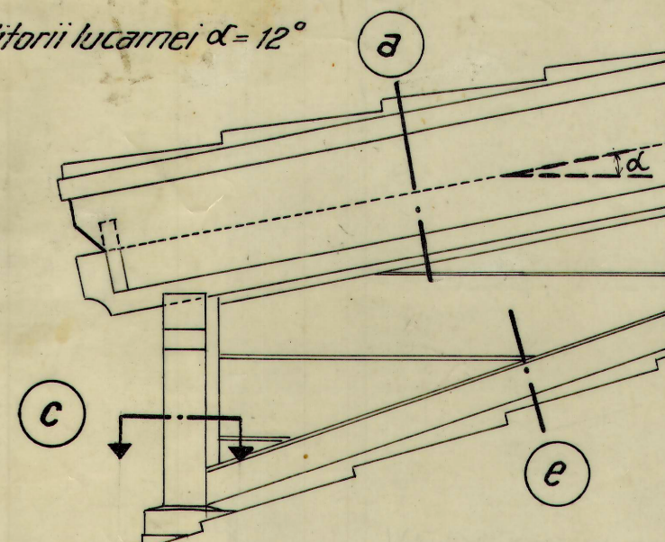
VEDERE LATERALĂ
